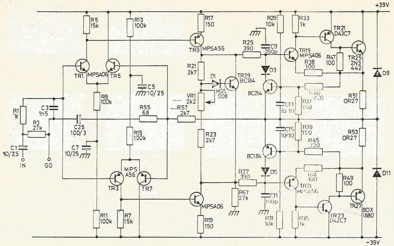
Lecson AP1. Schema elettrico « seconda versione » (vedi testo).
