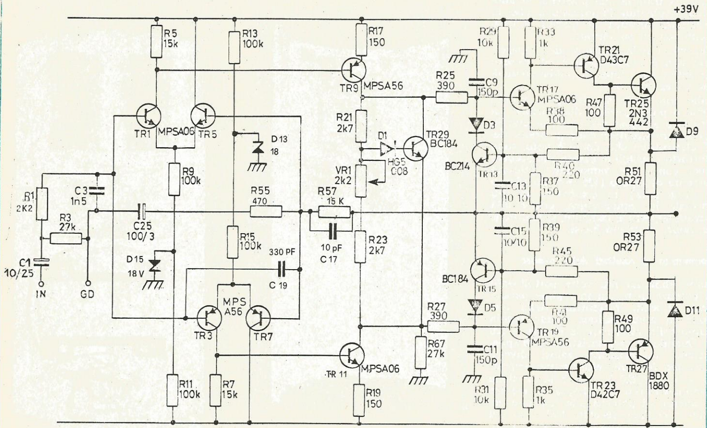
Lecson AP1. Schema elettrico « terza versione » (vedi testo).
